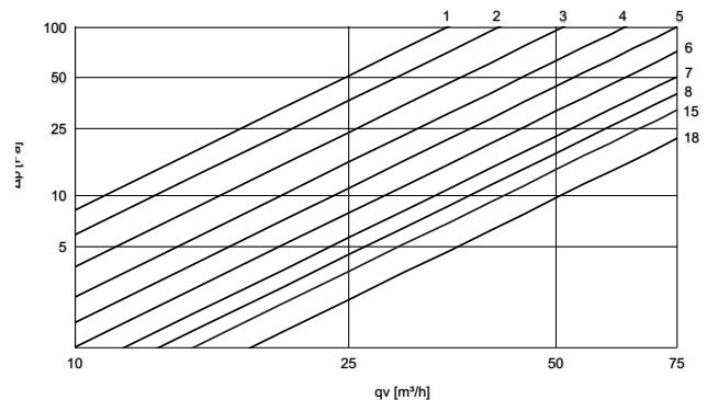
DRUKVERLIEZEN BIJ TOEVOER
