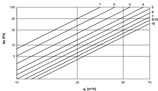
DRUKVERLIEZEN BIJ AFVOER
